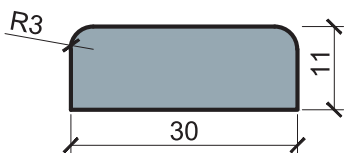
PI362
