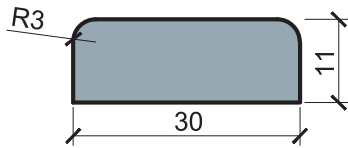
PI360
