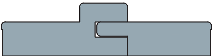
PI342 - 67X28mm
